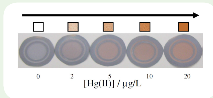
ภาพที่ 2 แผนภาพแสดงสีของแผ่นทดสอบที่ปริมาณปรอทแตกต่างกัน โดยทดสอบสารละลายตัวอย่างที่พีเอช 2
