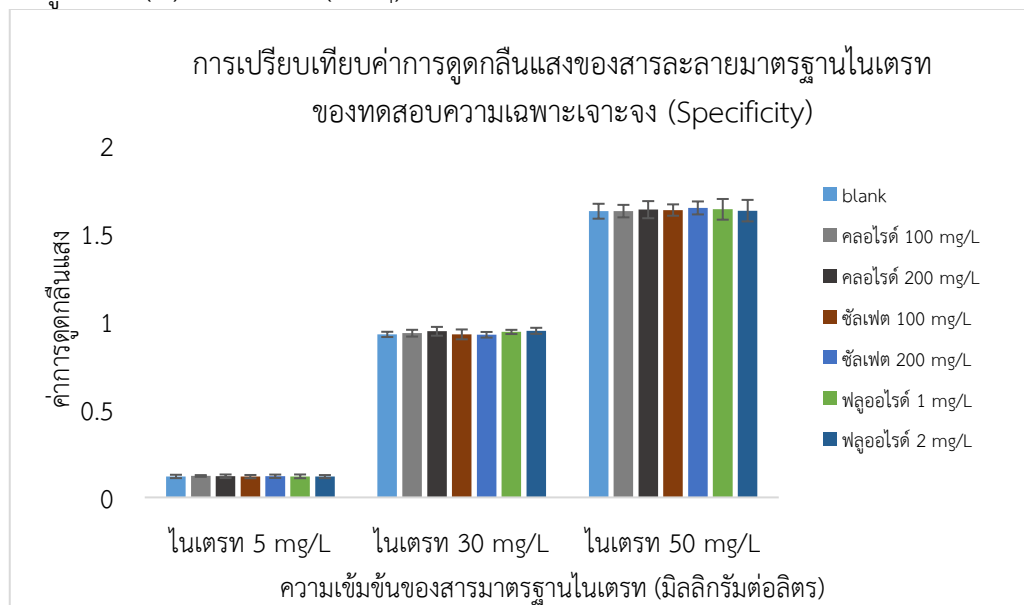
ภาพที่ 8 กราฟแสดงค่าการดูดกลืนแสงที่ 513 นาโนเมตรของสารมาตรฐานไนเตรท เมื่อมีไอออนของคลอไรด์ ซัลเฟต และฟลูออไรด์เป็นตัวรบกวน
