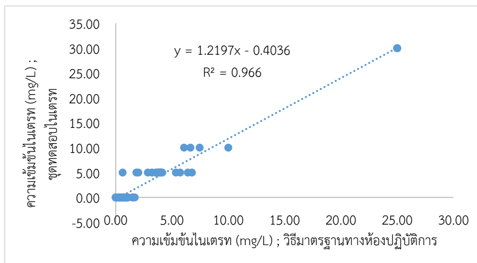
ภาพที่ 9 กราฟแสดงผลเปรียบเทียบการทดสอบไนเตรทด้วยวิธีมาตรฐานและชุดทดสอบไนเตรท
