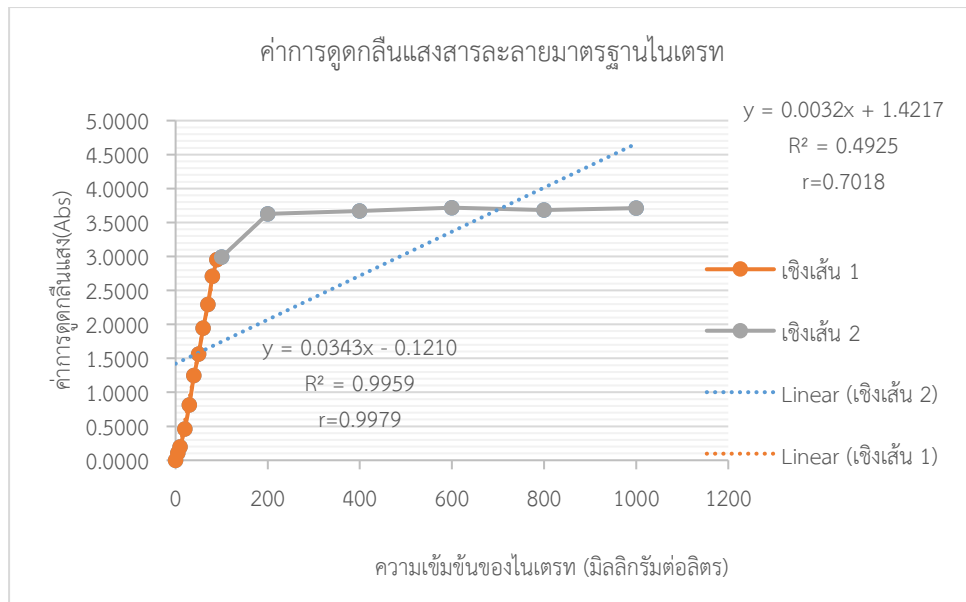
ภาพที่ 6 ความสัมพันธ์ระหว่างค่าการดูดกลืนแสงและความเข้มข้นไนเตรท ในการทดสอบความเป็นเส้นตรง (linearity)
